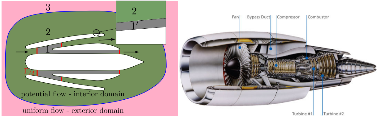
Fig. 1.4. Gauche : représentation schématique d'un turboréacteur, avec les trois zones de comportement identifiées (1,1' : écoulement complexe, 2 : écoulement potentiel, 3 : écoulement uniforme), droite : coupe réaliste d'un turboréacteur.
