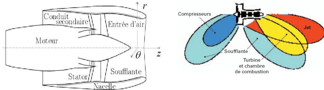
Fig. 1.2. Gauche : schéma d'une nacelle de turboréacteur (image issue de [40]), droite : principales composantes du bruit généré par un turboréacteur (image issue de [67]).
