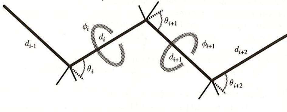
Figure 1.1 – Les interactions interatomiques dans une chaîne d’alcane: d_i désigne la distance entre deux atomes consécutifs, \theta_i est l’angle entre deux liaisons reliant trois atomes et \phi_i est l’angle dièdre qui sépare deux plans contenant chacun trois atomes. Image tirée de [Rapaport, 2004].
