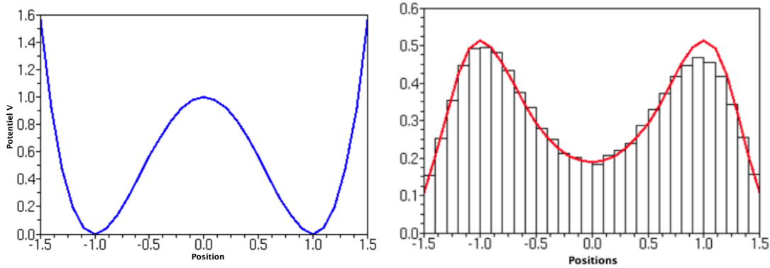
Figure 1.4 – Echantillonnage par la dynamique de Langevin amortie. Gauche: Le potentiel V(x) = (x^2 - 1)^2 . Droite: Distribution des positions après 10^5 pas de temps (barres verticales) et la mesure canonique associée à V (courbe rouge). Les paramètres utilisés: \beta = 1 et \Delta t = 0.001 .
