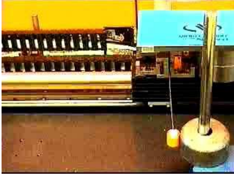
Figure 1: Simple masse reliée élastiquement à un moteur linéaire.
