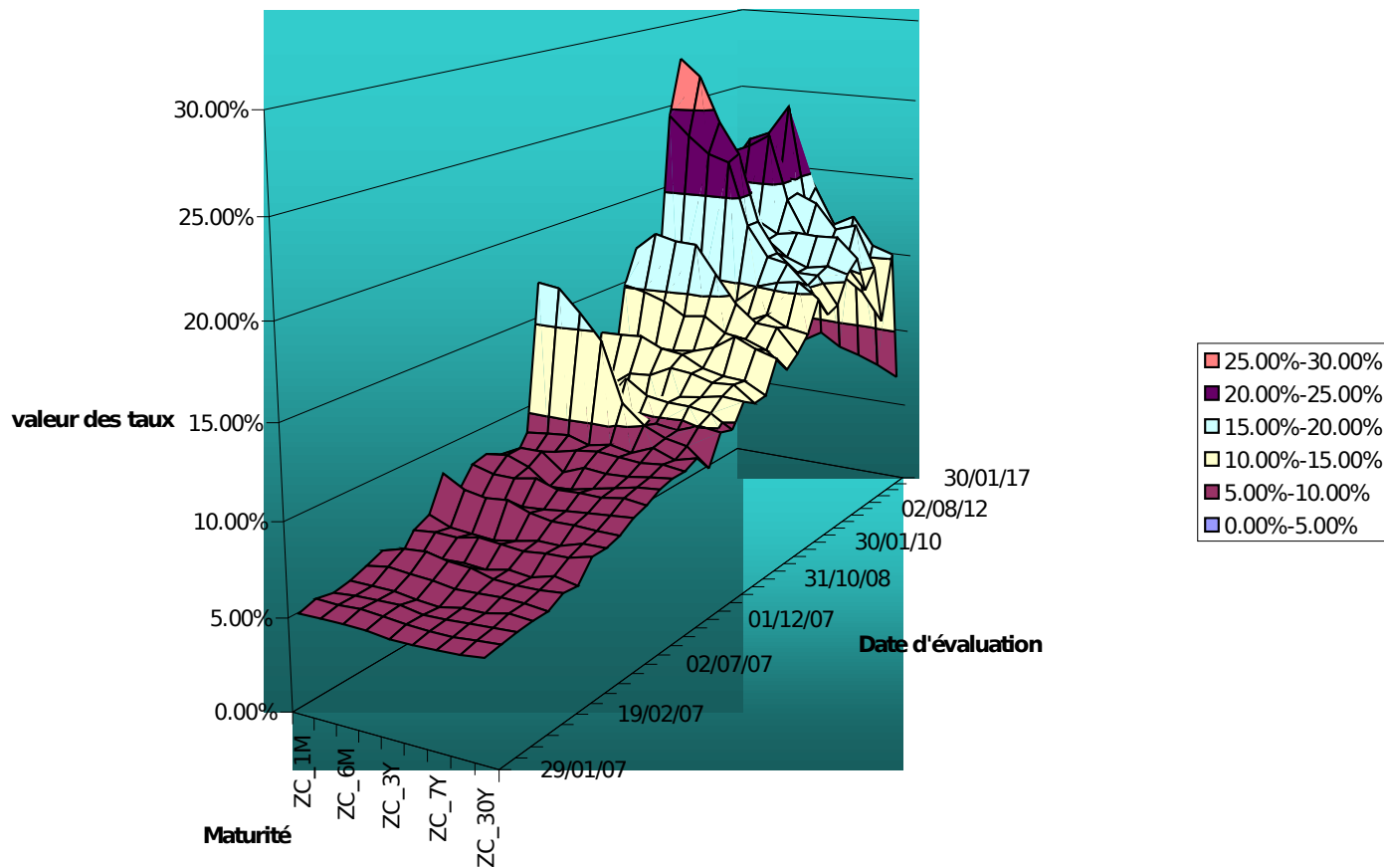
Scénarios de taux produisant l'exposition quantile
