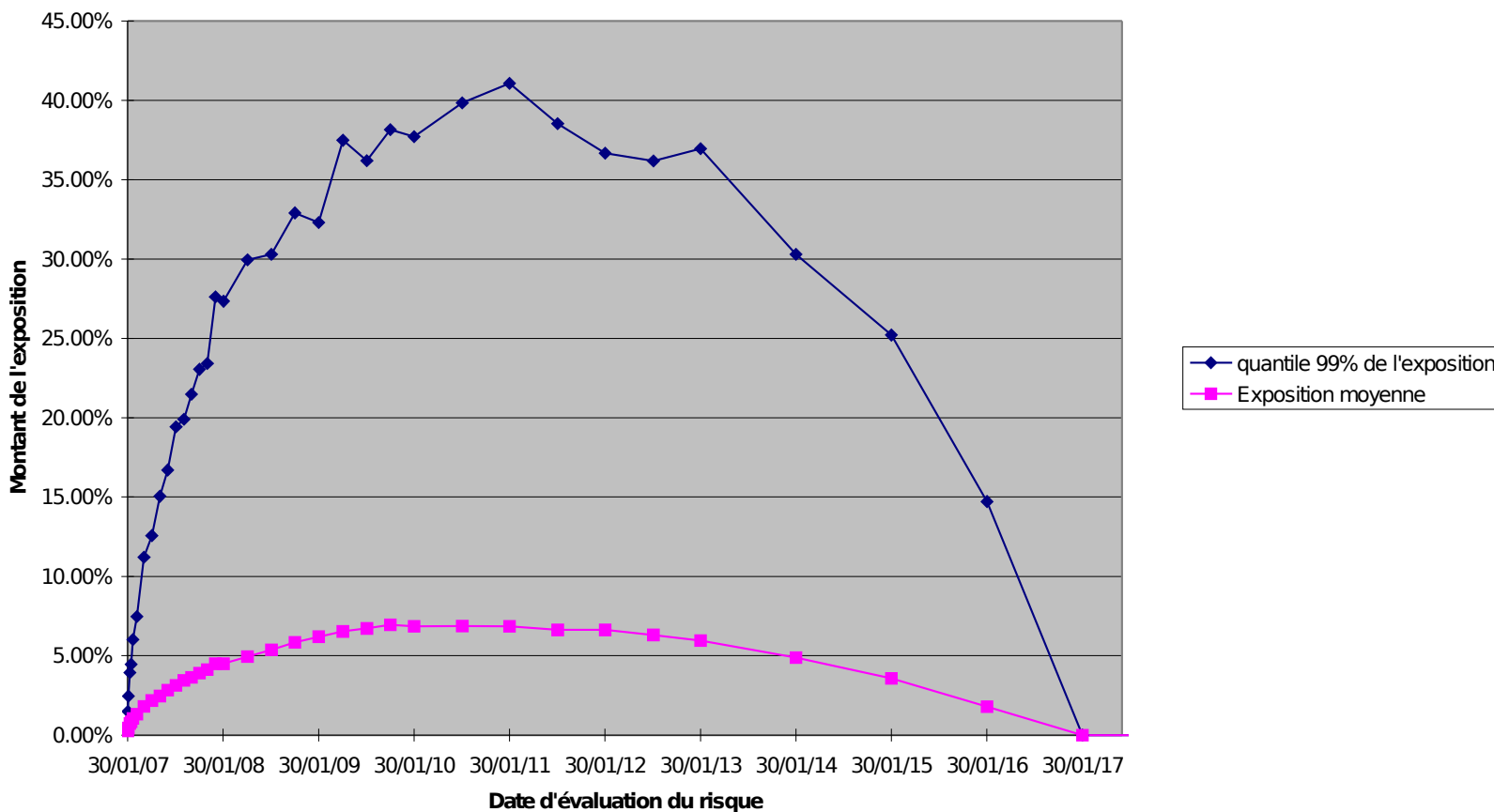
Profil de la CVAR d'un swap USD/LIB 6M maturité 10Y
