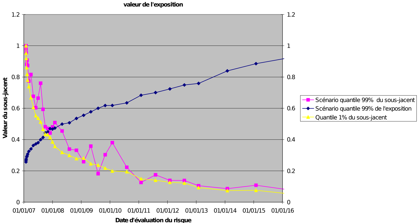
Profil de la CVAR d'un Put à la monnaie vol histo 40% cost of carry 4%
