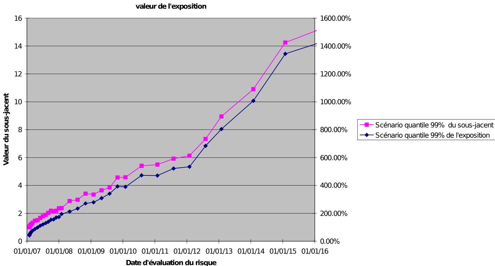
Profil de la CVAR d'un Forward à la monnaie vol histo 40%
