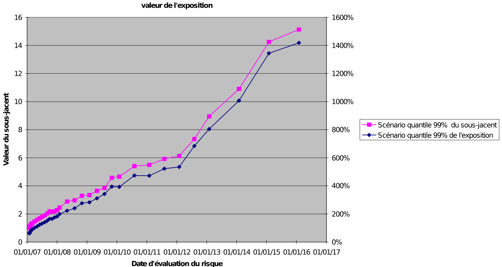
Profil de la CVAR d'un call à la monnaie vol histo 40%
