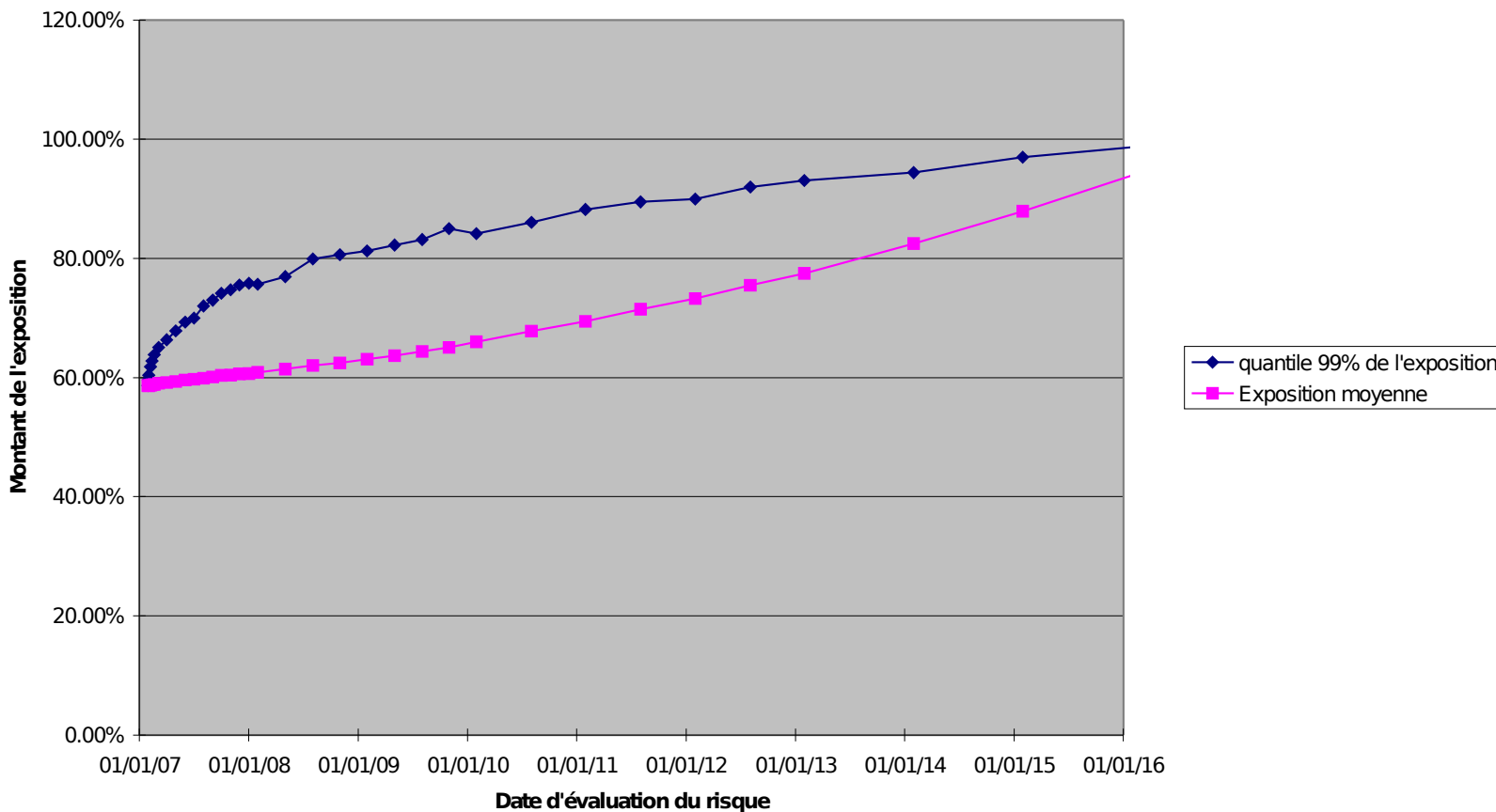
Profil de la CVAR ZC USD
